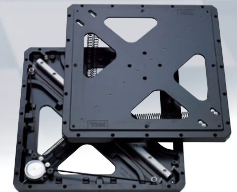
重荷重対応・床免震対応 免震モジュールTGS型
